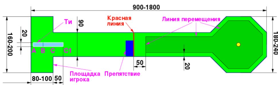
Рисунок 4. Основные размеры и разметка дорожки стандарта «фетровый мини-гольф»
