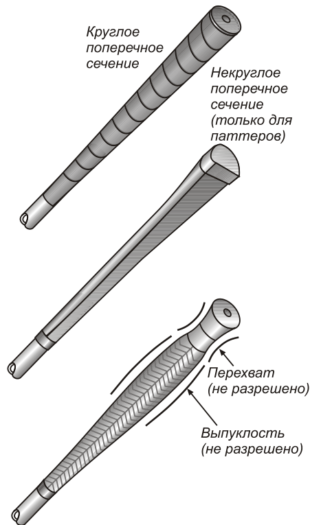
Рисунок 11. Требования к рукоятке
