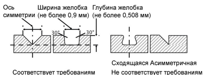
Рисунок 15. Требования к форме желобков
