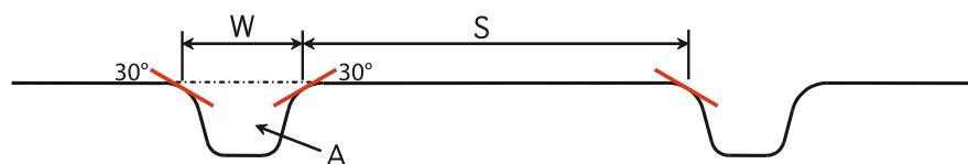
Рисунок 16. Ширина и шаг желобков
