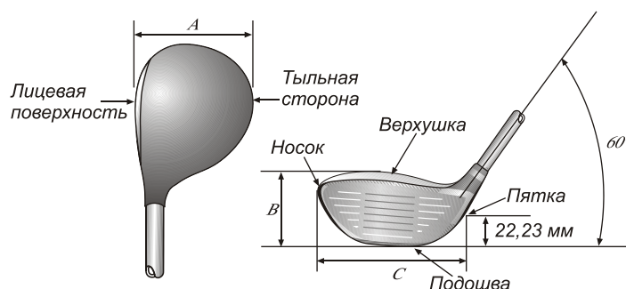
Рисунок 12. Измерение головки вуда
