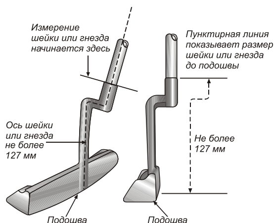
Рисунок 10. Измерение длины шейки
